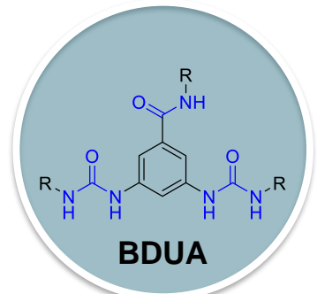
benzene diurea monoamide
