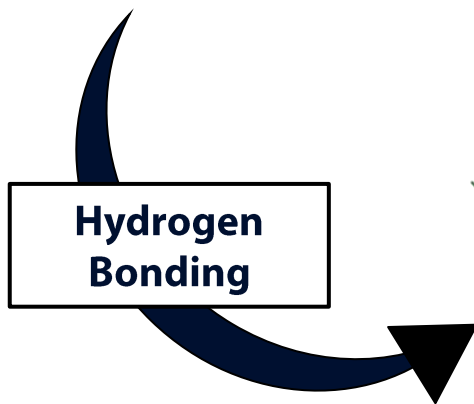
benzene diurea monoamide
